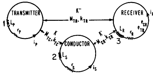
Figure 7.6. Electric-circuit analogy for EM system.
